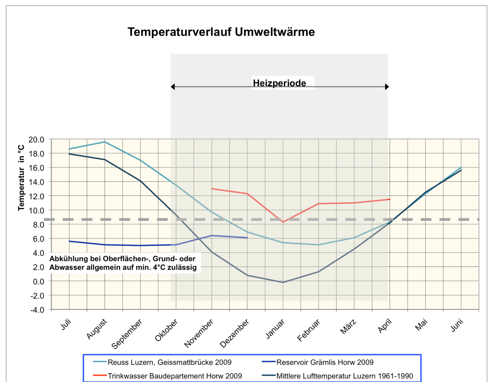
Abb. 12: Temperaturverlauf verfügbarer Umwelt- und Abwärmequellen (Quelle: MeteoSchweiz, BAFU, eigene Darstellung)
