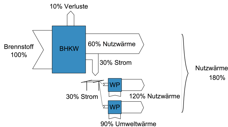
Abb. 15: Prinzipskizze und Nutzungsgrad einer wärmegeführten WKK-Anlage (Quelle: PLANAR)
