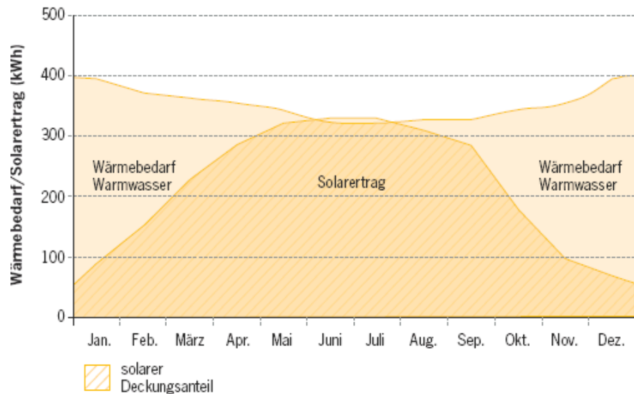
Abb. 13: Wärmebedarf zur Warmwasseraufbereitung (für 5 Personen und 5 m 2 Flachkollektoren) im Jahresverlauf 30
