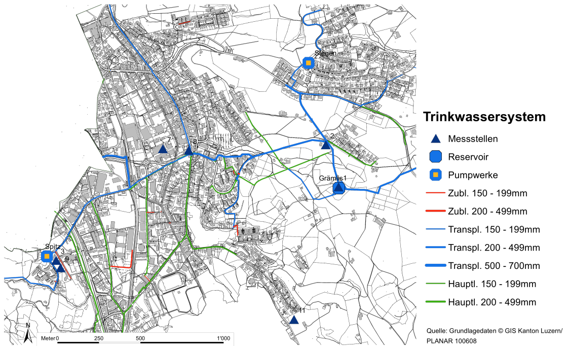
Abb. 9: Trinkwassersystem (Pumpwerke, Reservoirs, Leitungen, Temperaturmessstellen); vgl. Anhang
