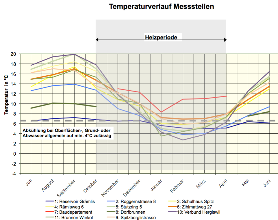
Abb. 10: Temperaturverlauf Trinkwassermessstellen 2009
