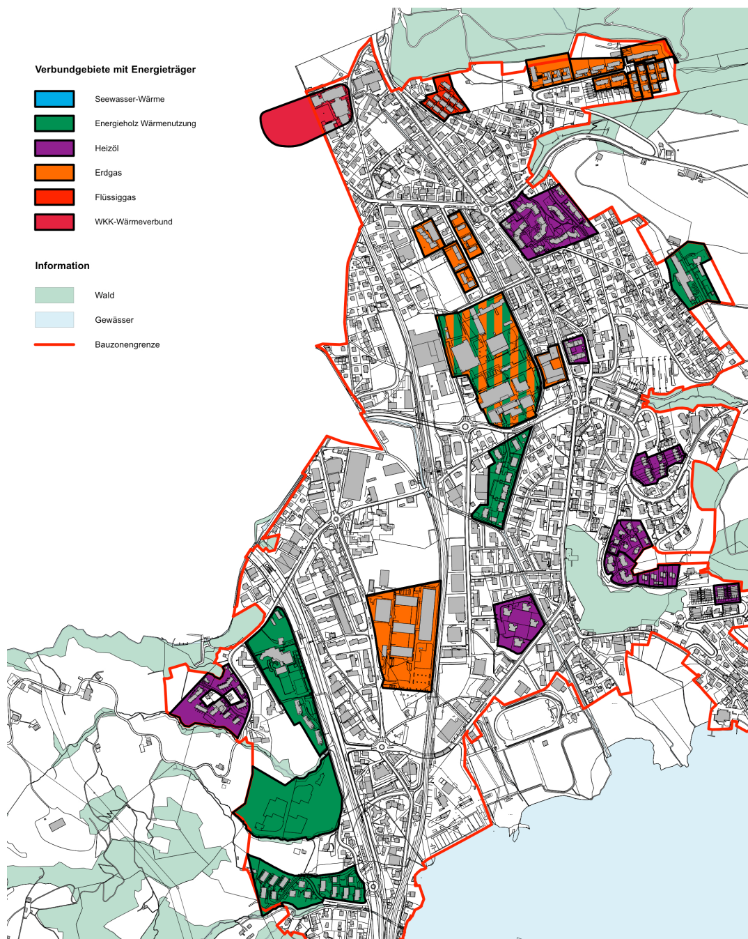
Abb. 5: Bestehende Wärmeverbunde im Ortszentrum
