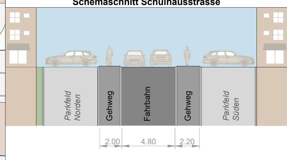
Schemaschnitt Schulhausstrasse
