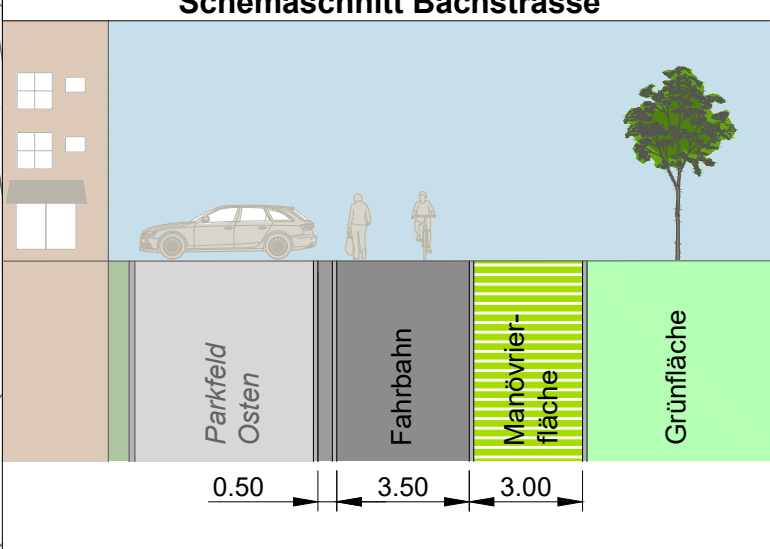
Schemaschnitt Bachstrasse
