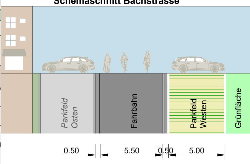
Schemaschnitt Bachstrasse
