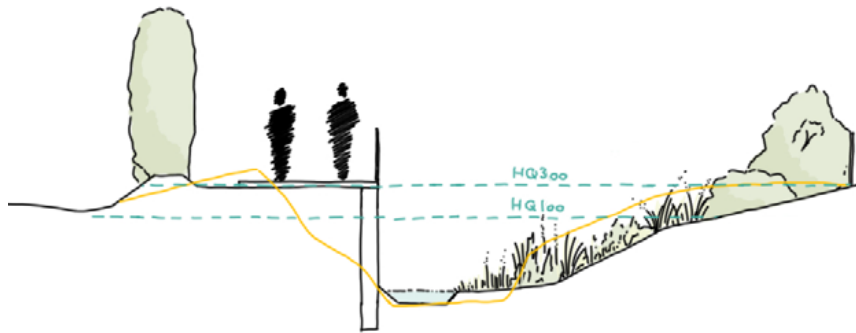
Querschnitt Dorfbach Weg bachaufwärts
