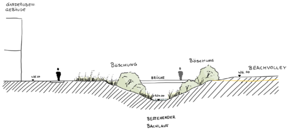
Querschnitt Sportplatz- bach Sportachse
